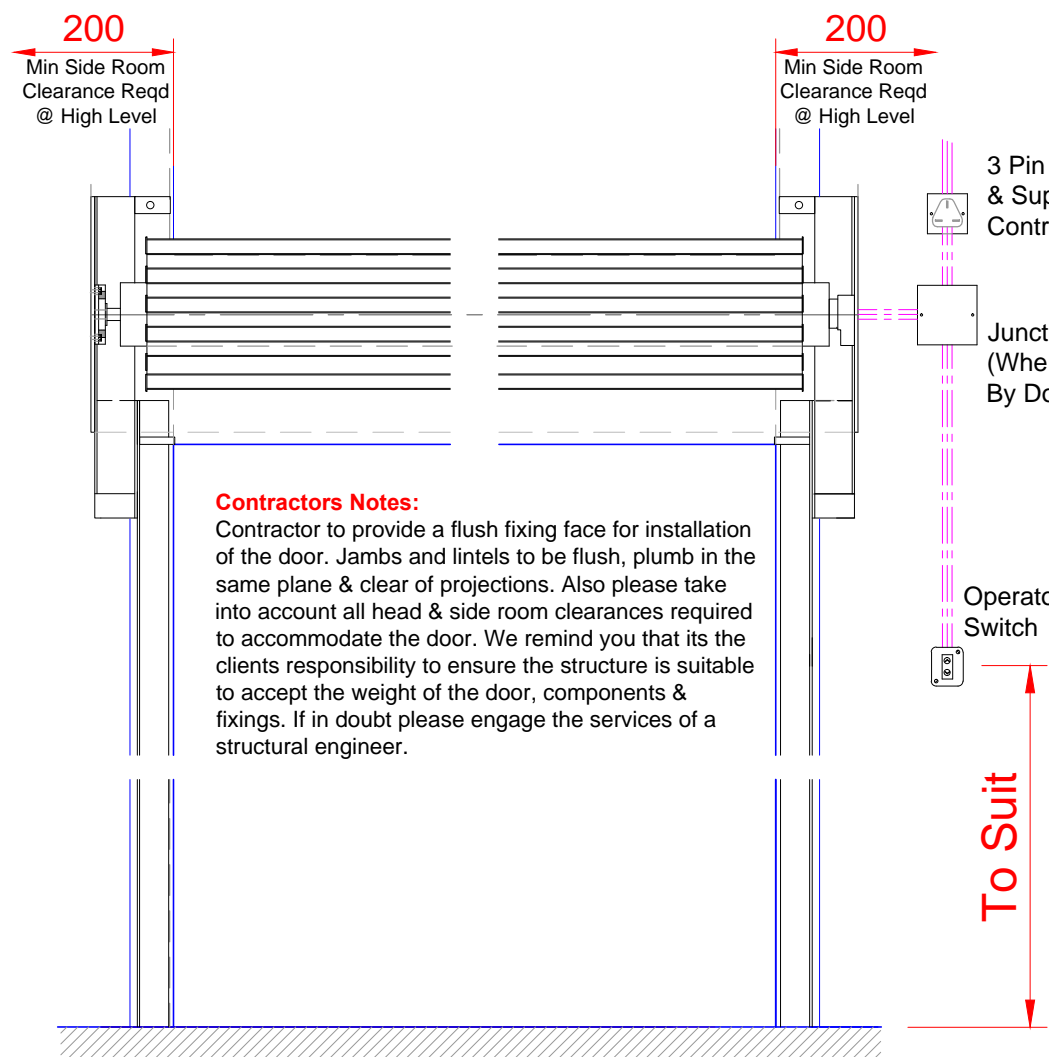
ELEVATION
